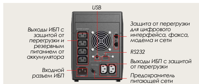
Protect A. 1000 / A. 1400 – вид сзади
