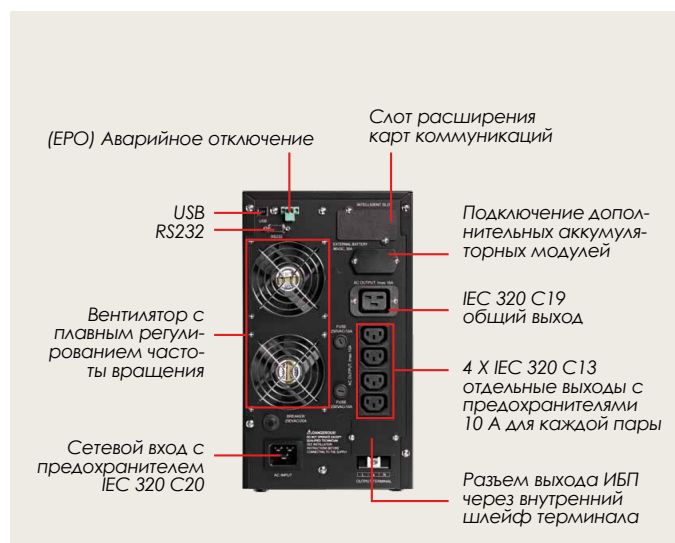
Protect C. 3000 – вид сзади
