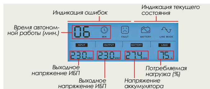
Protect A. 1000 / A. 1400 – дисплей
