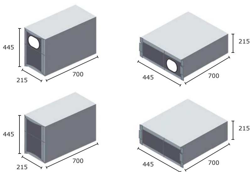
Габаритные размеры Solo MD
