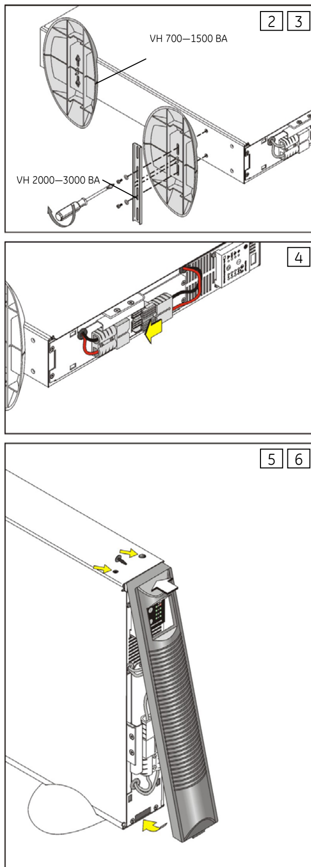
Рис. 3.3.1: Подготовка к вертикальной установке
