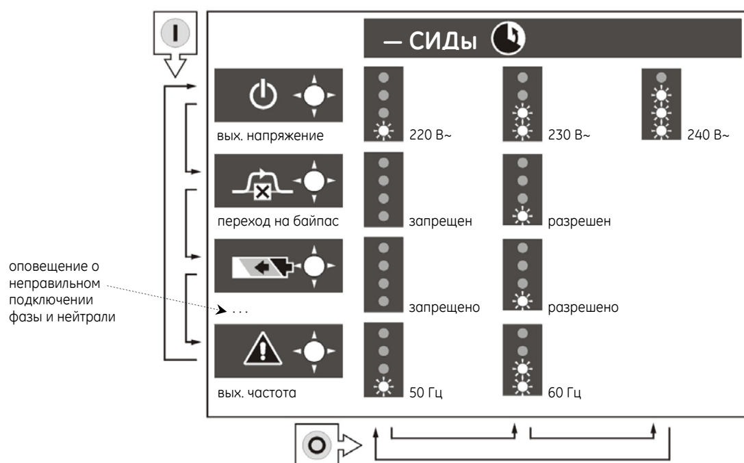
Рис. 4.5: Меню настройки
