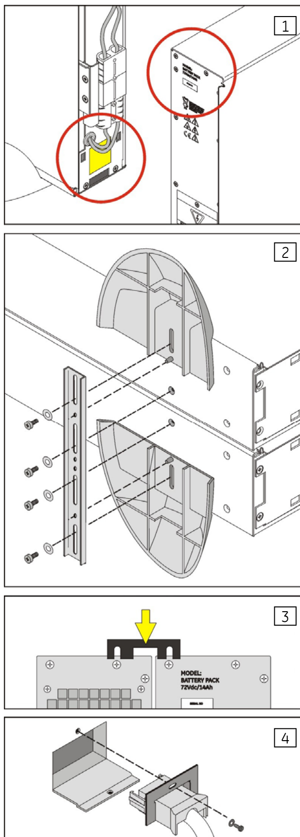
Рис. 3.3.4а: Установка дополнительных батарейных блоков и подключение их к ИБП
