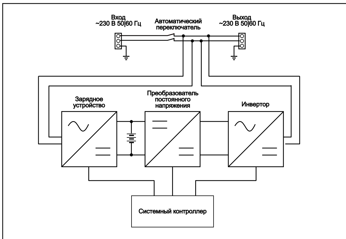
ОБЩАЯ ФУНКЦИОНАЛЬНАЯ СХЕМА
