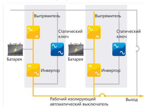
Параллельная конфигурация с распределённым байпасом
