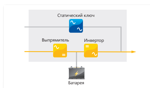
Моноблочная конфигурация
