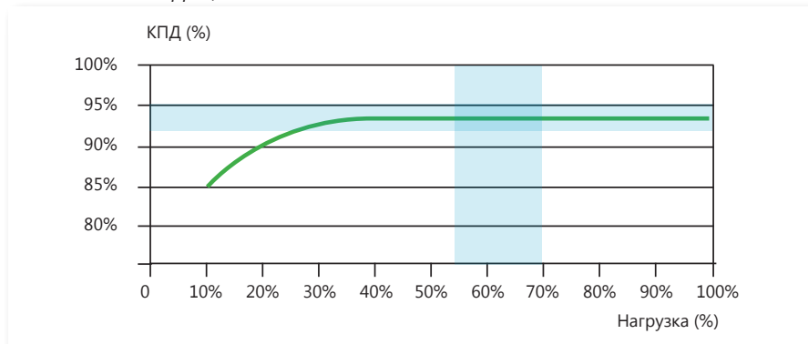
Liebert® NXL 400кВА - КПД в режиме двойного преобразования
