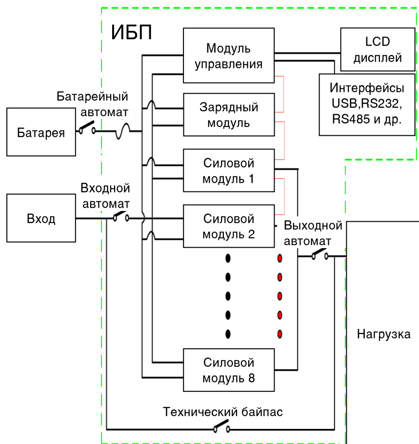
Структура ИБП EA660 160 кВА
