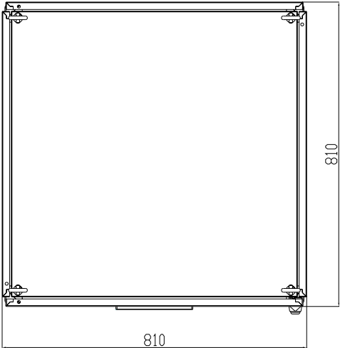
Модель ONL- II-45K/60K33 120В/208В и ONL - II-45~120K33 220В/380В
