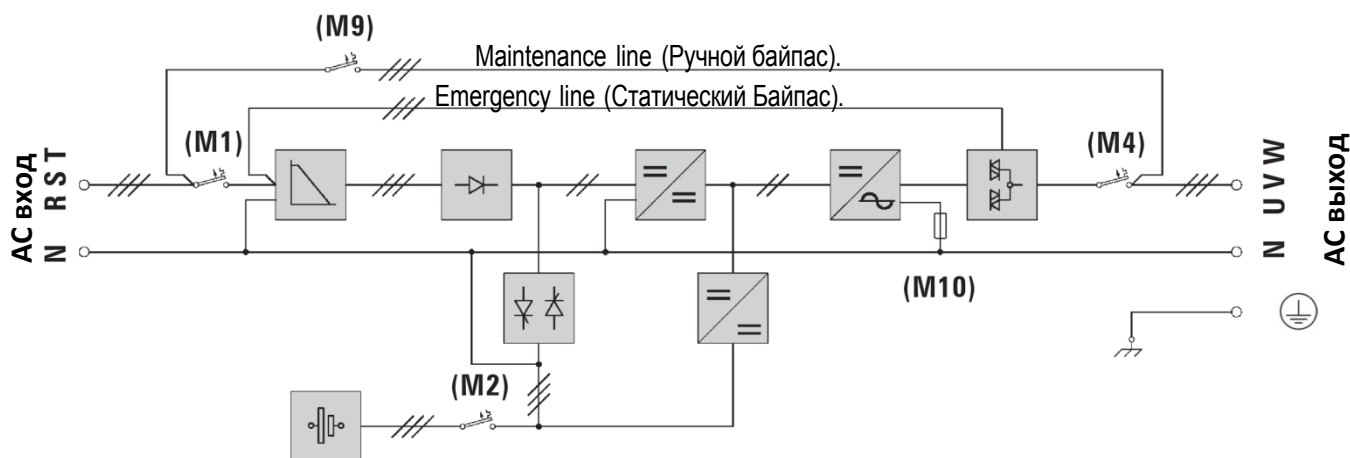
Рис.1.1 VGD33 блок-схема.
