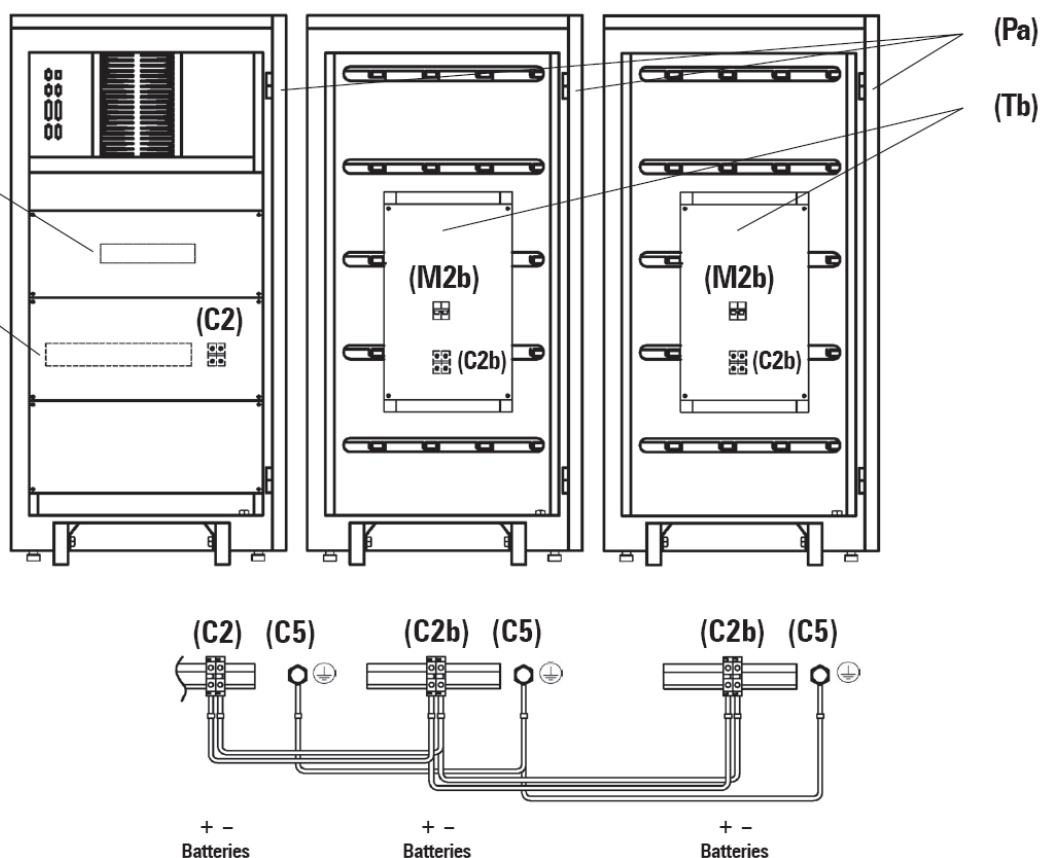
Рис. 12. Соединение между ИБП и 2 батарейными кабинетами.
