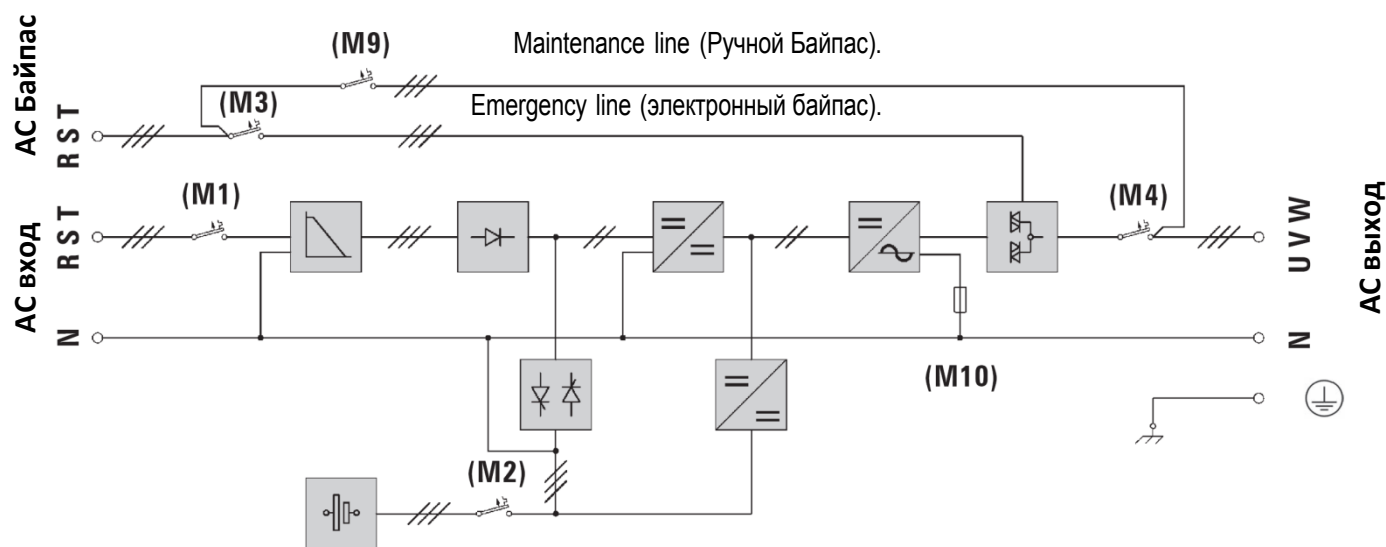
Рис.1.2 VGD33-B блок-схема.
