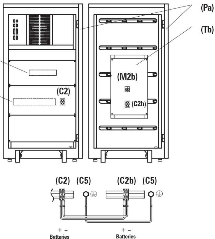
Рис. 11. Соединения между ИБП и батарейным кабинетом.
