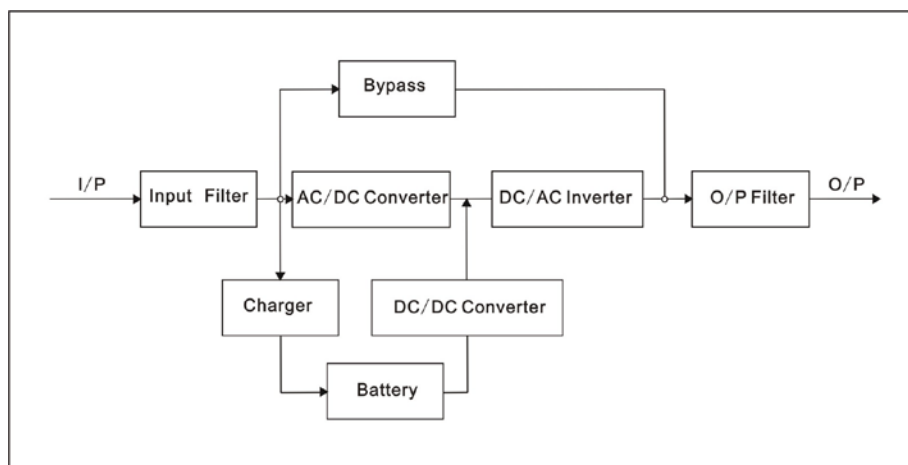
Рис.1 Блок-схема ИБП
