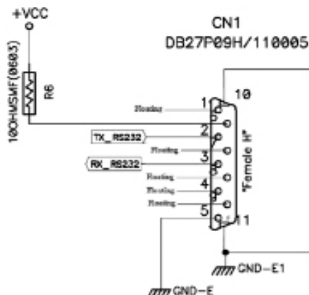
Порт RS 232
