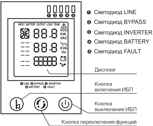
Рис. 1 Передняя панель блока ИБП
